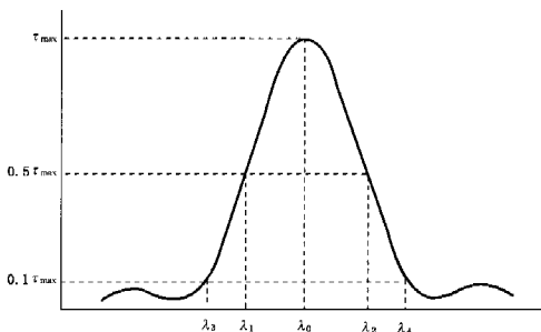
图 1 波长-透射比光谱曲线
